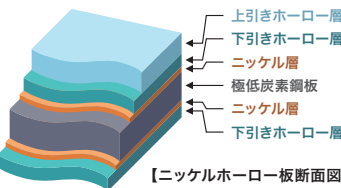
【ニッケルホーロー板断面図】
